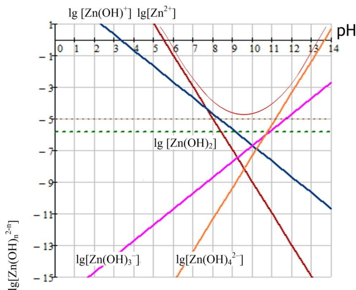
Рис. 4 – Утворення гідросокомплексів цинку
