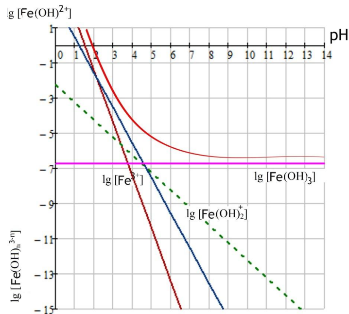
Рис. 3 – Утворення гідросокомплексів феруму (III)
